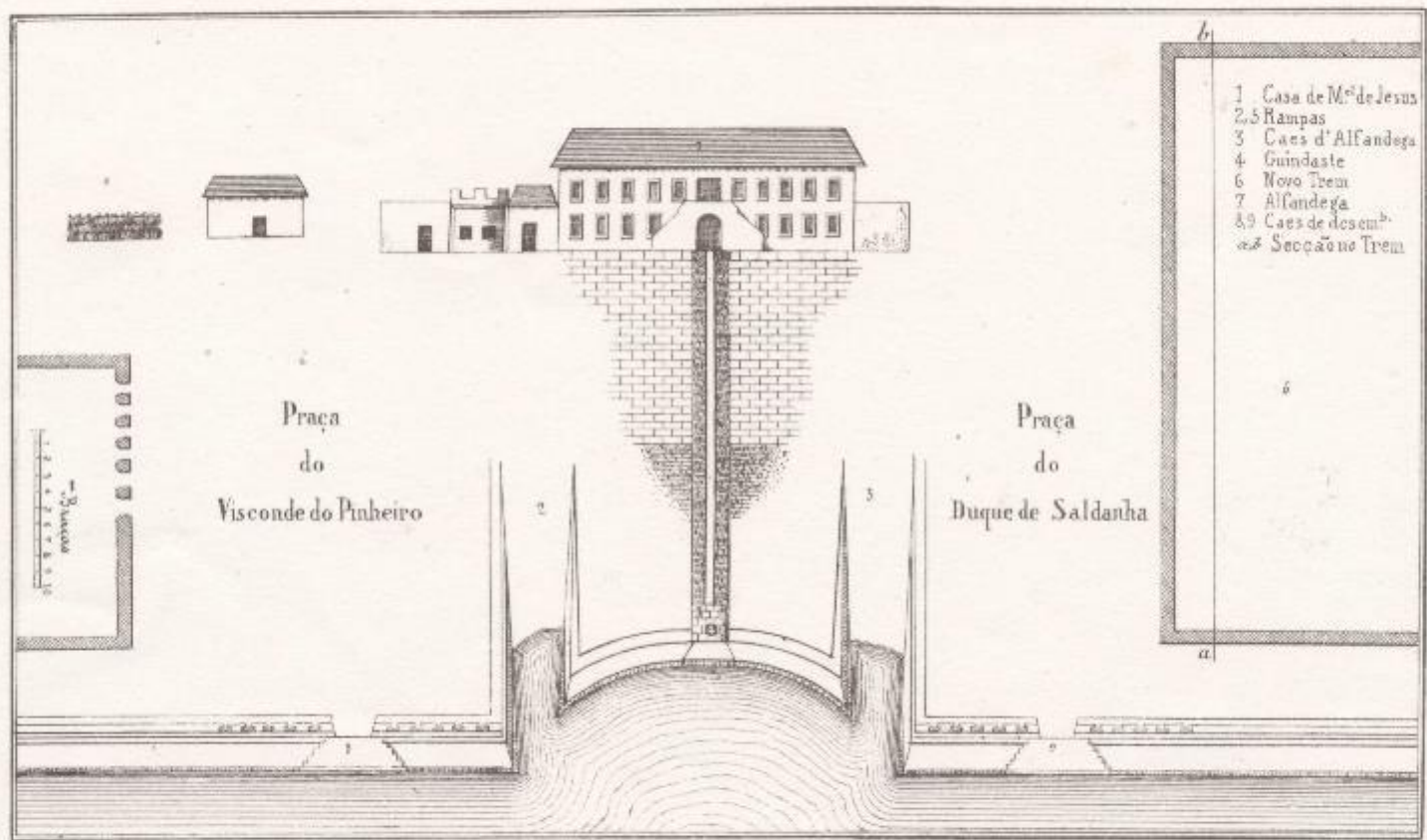
PLANTA DAS OBRAS NO CAES DA ALFANDEGA DE LOANDA MANDADAS FAZER PELO GOVERNADOR GERAL VISCONDE DO PINHEIRO
